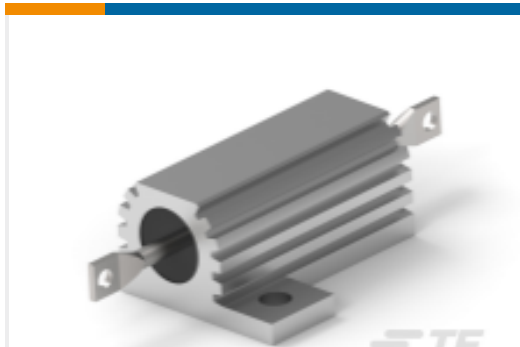
TE 产品编号1-1879075-4 功率电阻器：铝壳体，75 瓦特
