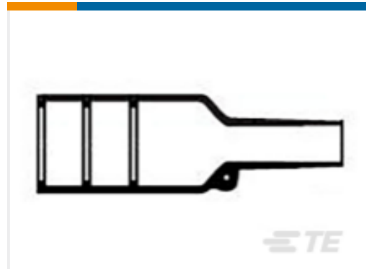
TE 产品编号878496-000 球形热缩护套：有嘴，直形
