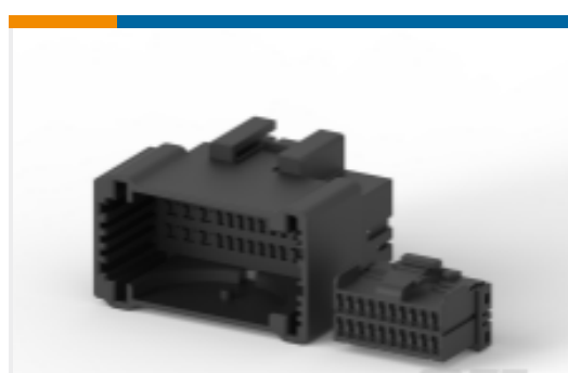
TE 产品编号917975-1 MULTILOCK, 连接器壳体
