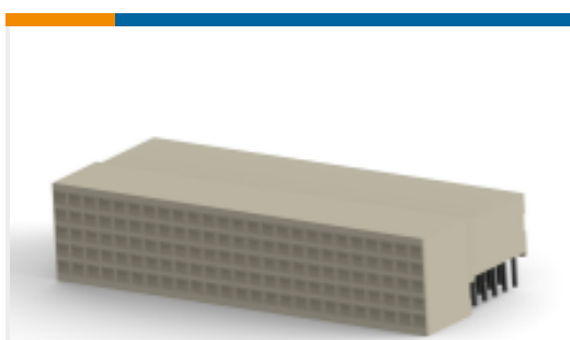
TE 产品编号1857994-1 HM 插座连接器：传统背板，共面，2mm
