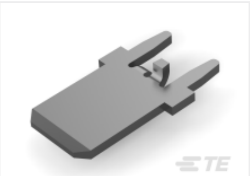
TE 产品编号1742188-1 250 FASTON,PCB TAB,TCBR
