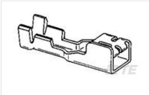
TE 产品编号142686-1 L.I.F PL CONTACT 5MM 1 TO 3 MM2 PTPPHBZ
