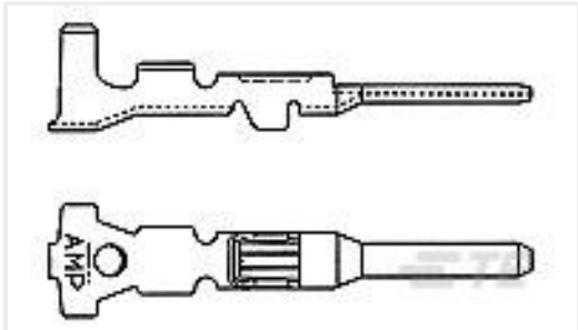
TE 产品编号282109-3 MINI MIC TAB CONTACT
