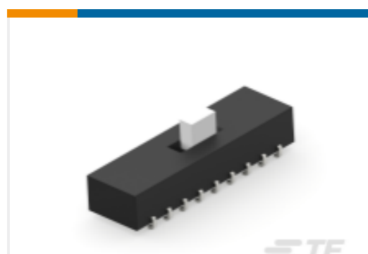
TE 产品编号 4-1825010-4 ASE62S04=6PDT AUTOSLIDE
