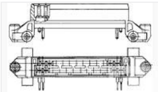
TE 产品编号1-794223-0 MINI UMN2 SCKT 20-16AWG 30AU
