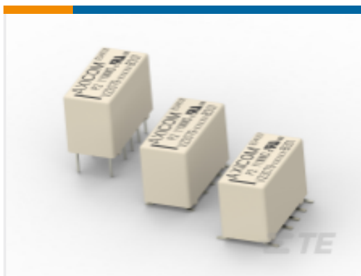
TE 系列/零件编号3-1393788-5 AXICOM P2 标准
