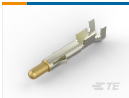
TE 产品编号 350547-6 UMNL PIN 20-14 AU/PHBZ L/P
