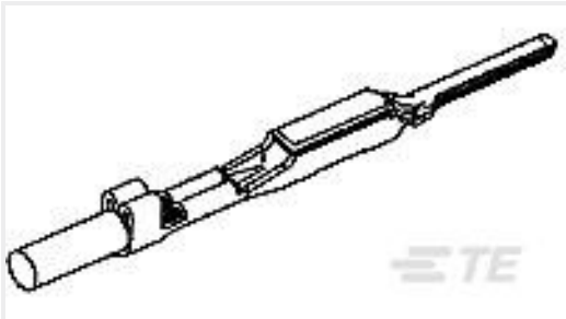
TE 产品编号353537-1 040-3 UNSEALED CONT. TAB(S)
