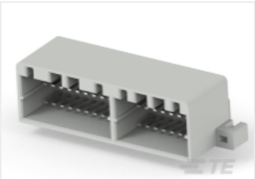
TE 产品编号 179059-7 040 MLC MK-2 CAP ASSY 36P
