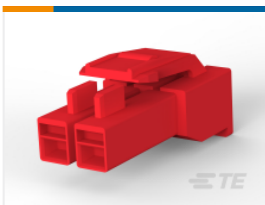
TE 产品编号 176271-2 AMP UNIVERSAL POWER PLUG 2P
