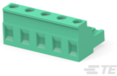
TE 产品编号 796981-5 5 POS TERMI-BLOK R/A PLUG 7.62
