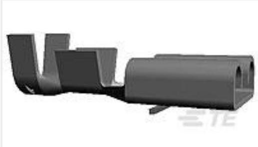
TE 产品编号170089-1 FF 250 REC 14-12AWG BR
