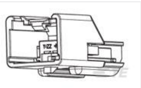
TE 产品编号6-1419166-1 1X4MALE IL ASSY "A"
