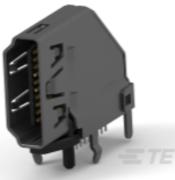
TE 产品编号 2007435-1 Std HDMI, Flag, T/H
