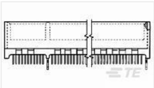
TE 产品编号 1734774-1 PCI EXP 3.1L 36 POS WHT G/F
