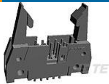
TE 产品编号5499206-4 A/L UNIV HDR 20P VERT LG LAT
