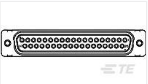
TE 产品编号1484950-1 AMPLIMITE PLG ASY,25P,SZ3,SER109
