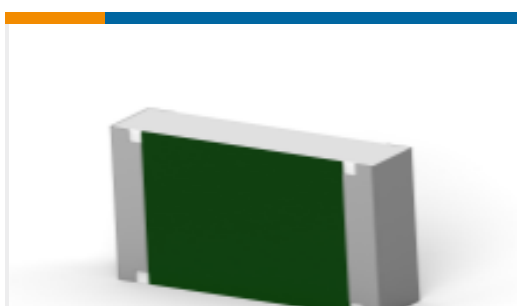
TE 产品编号 5-2176397-0 3502 110R 1%
