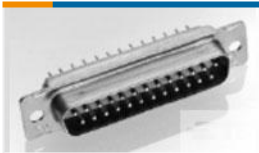
TE 产品编号 204505-1 AMPLIMITE,ASY,PLUG,STD,90,3
