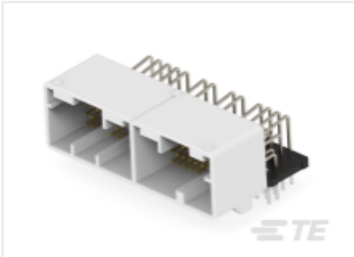
TE 产品编号1473193-5 025/040 CAP HSG ASSY 70P
