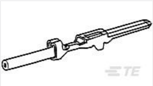
TE 产品编号173645-3 070 MLC TAB CONT 20-16 GOLD
