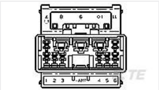
TE 产品编号174942-1 070 MLC W-W CAP HSG 15P
