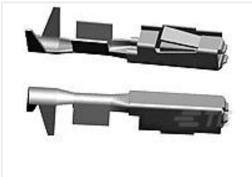
TE 产品编号968075-2 MPQ2,8 Sn rec LL unseal. >1-2,5
