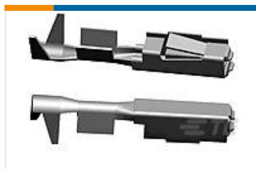
TE 产品编号5-968221-6 MQS0,63 Ag rec CB unseal. 0,5-0,75
