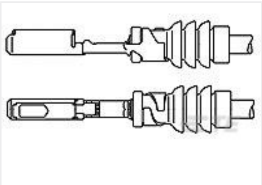
TE 产品编号1703032-1 MQS0,63 Sn rec CB EDS 0,5-0,75
