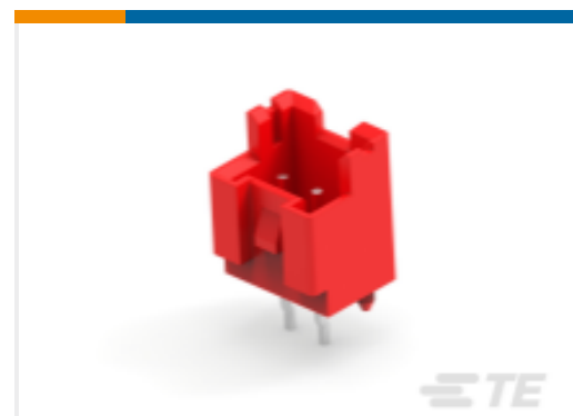
TE 产品编号2338245-2 EP2.5 HDR 2P VERT BOSS,RED,UL
