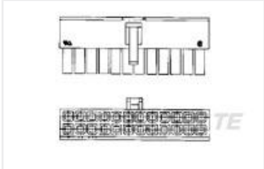
TE 产品编号1-794954-8 18P RCPT VAL-U-LOK V2
