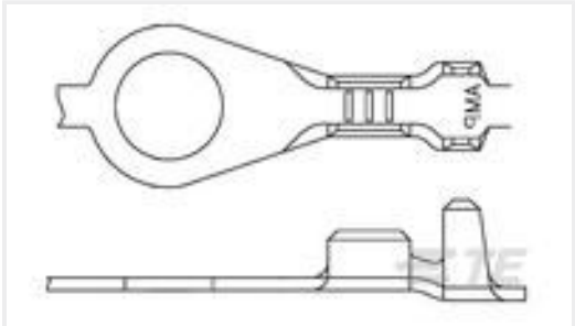
TE 产品编号880665-2 RING TONGUE
