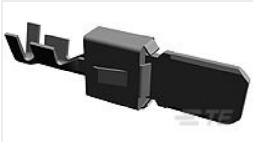
TE 产品编号964306-1 TAB A 5.8x0.8 CONTACT CF SRC Sn
