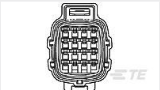
TE 产品编号368047-1 E-S MK-2(+) 16P PLUG ASSY
