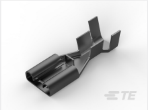
TE 产品编号 1217095-2 RCPT 250 POS-LOCK 16-12 TPBR
