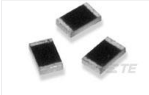
TE 产品编号9-1879256-5 RP 2B 237R 0.1% 15PPM 1K RL
