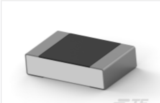
TE 产品编号9-2176374-8 RQ 0805 1K1 0.1% 10PPM 1K RL
