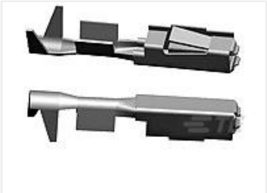
TE 产品编号1355717-1 MQS0,63 Sn rec LL unseal. 0,08-0,22
