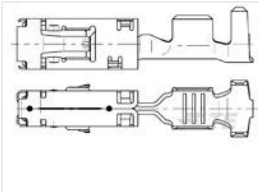
TE 产品编号967541-1 2.8MM SENS FLA-KONT
