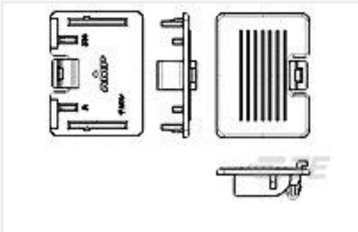
TE 产品编号1-1123919-4 1.5 MINI CT DUST COVER
