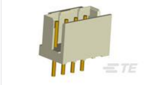
TE 产品编号 CAT-3984552-PHITPS CT 柱板端连接器组件：Part.带罩
