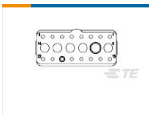
TE 产品编号1738151-1 Insert Asy,Pin,Arr 22,Environ,Key B
