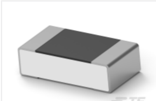
TE 产品编号2176371-3 RQ 0603 4K87 0.1% 10PPM 5K RL
