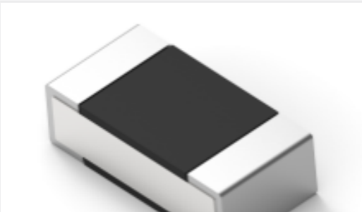
TE 产品编号7-2176307-1 RP 1E 0.1W 66K5 0.1% 25PPM 5K RL
