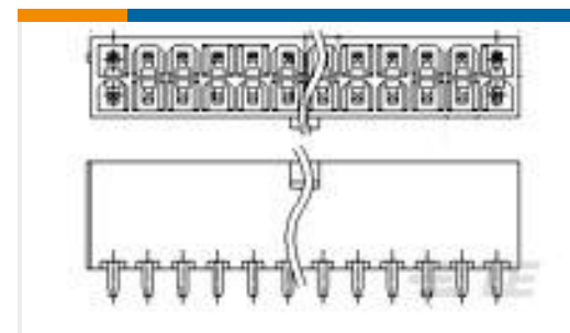
TE 产品编号4-1775099-6 ATX PWR CONN 18 POS
