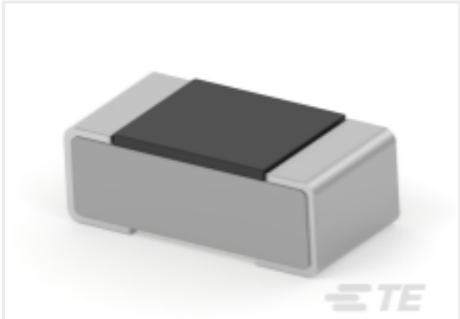
TE 产品编号2176338-1 CRGCQ 0402 1R0 5%
