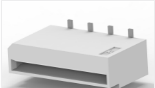
TE 产品编号 84982-8 1MM FFC SMT V ASSY 8P EMBOSS
