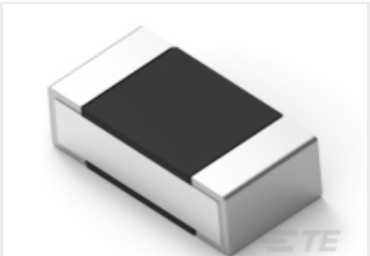
TE 产品编号9-2176307-8 RP 1E 0.1W 127K 0.1% 25PPM 5K RL
