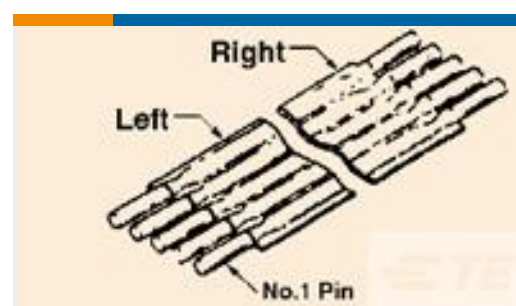
TE 产品编号7-1437142-2 FSN-22A-8=NOMEX FS STD
