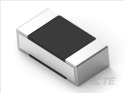
TE 产品编号4-2176306-9 RP 1E 0.1W 3K65 0.1% 25PPM 5K RL
