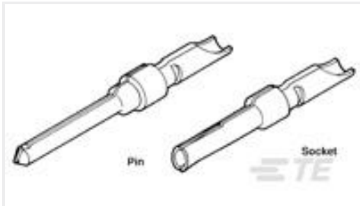
TE 产品编号1-66569-0 20 DF SOCKET CONT, SMALL PACK
