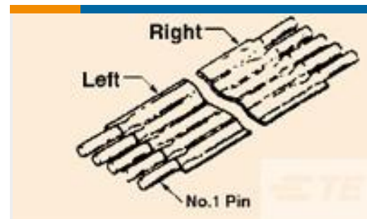
TE 产品编号3-1437130-3 FSN-11A-5=NOMEX FS STD
