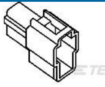
TE 产品编号172129-1 250 FASTON HSG, CAP 2P NATURAL
