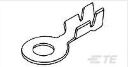
TE 产品编号62638-1 RING TONGUE 22-20 AWG TPBR
