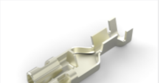
TE 产品编号2238104-1 250 PL MKII REC. 16-14AWG NPST
