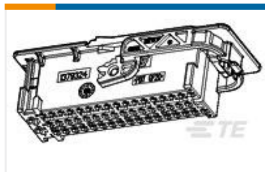
TE 产品编号1379324-1 52W HYB REC HSG ASSY BLAC
