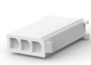
TE 产品编号 172344-1 MINI UNIVERSAL MATE-N-LOK CAP HOUSING 3P
