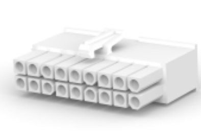
TE 产品编号 770584-1 18P MINI UMNL PLUG HSG
