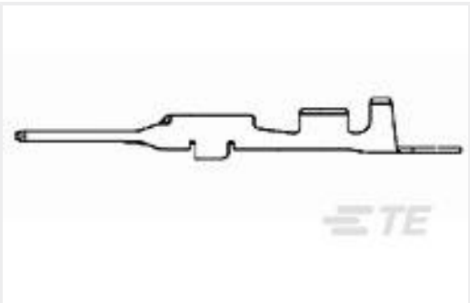
TE 产品编号1565963-1 040III TAB NON SEALED TIN
